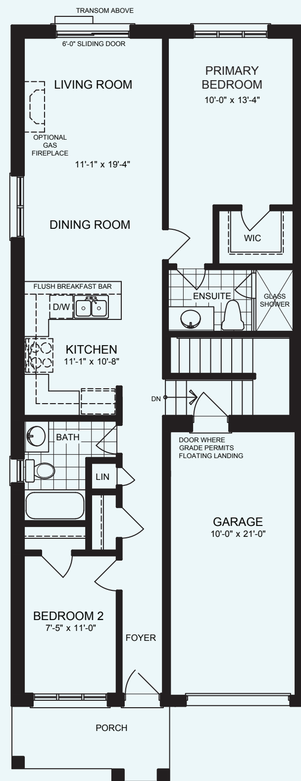
OPTIONAL MAIN LEVEL ELEV 'A' & 'B'
