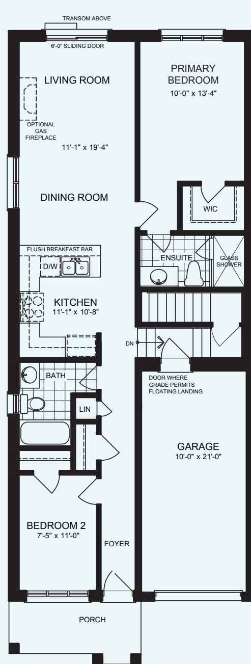
OPTIONAL MAIN LEVEL ELEV 'A' & 'B'
